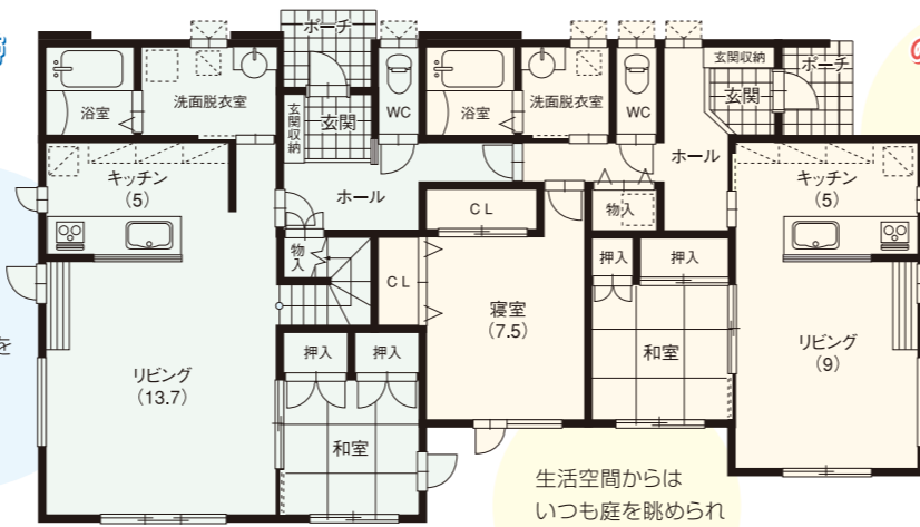
●1階床面積/132.49㎡ (40.00坪)
